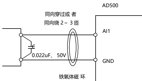
图 3-7 模拟量输入端子接线示意图
