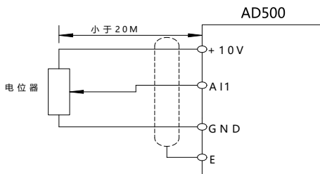
图 3-7 模拟量输入端子接线示意图
