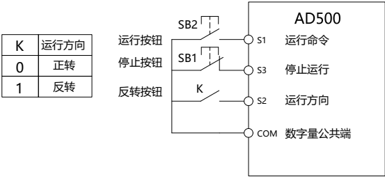
图 6-11 三线式控制模式 2
