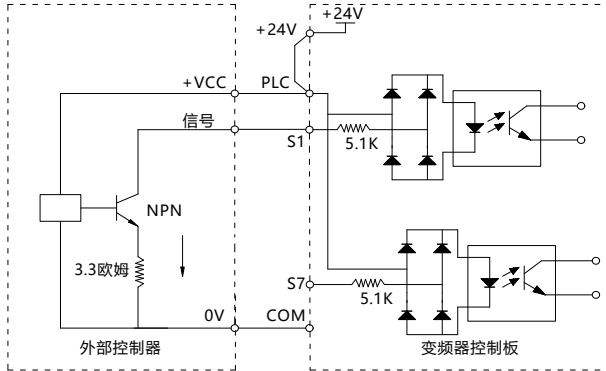
图 3-9 漏型接线方式
