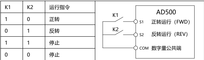
图 6-8 两线式模式 1
