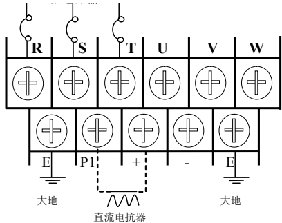
g) 132KW-315KW 变频器主回路端子台配线图 (如图 3-3g)
