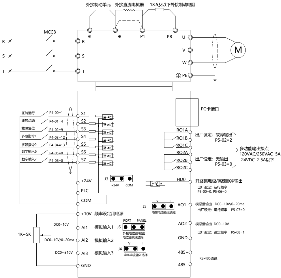
图 3-5 标准接线图
