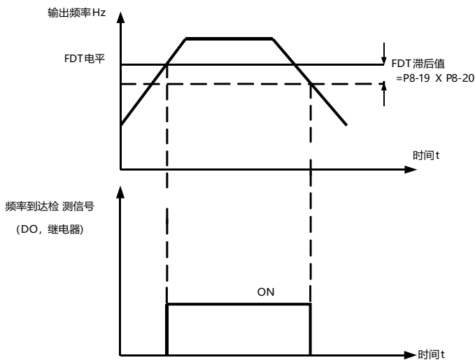
图 6-16 FDT 电平示意图
