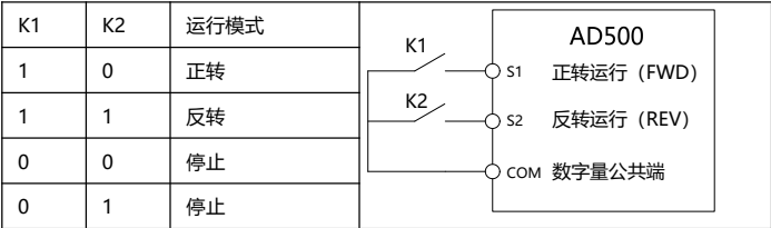
图 6-9 两线式模式 2
