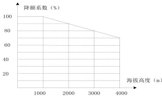
图 1-5 变频器海拔高度降额曲线图
