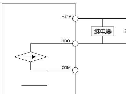
图 3-12 字输出端子接线示意图
