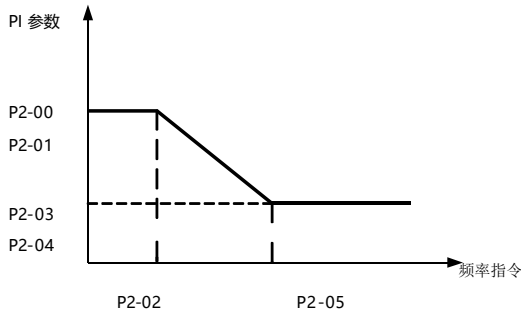
图 6-4 PI 参数示意图
