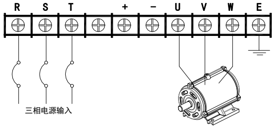
d) 22KW-30KW 变频器主回路端子台配线图 (如图 3-3d)
