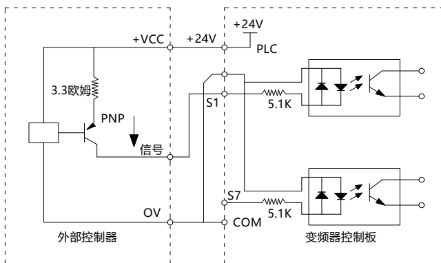
图 3-11 源型接线方式
