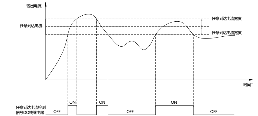
图 6-23 任意到达电流检测示意图
