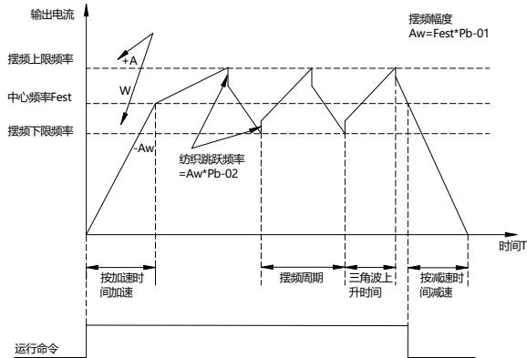
图 6-28 摆频工作示意图
