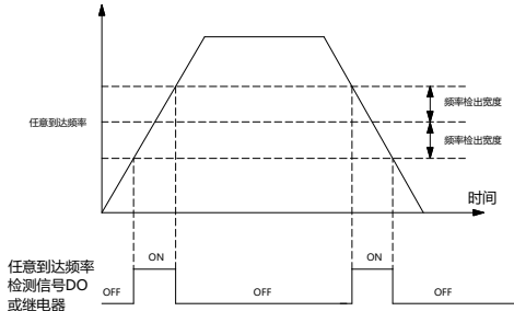
图 6-20 任意到达频率检测示意图
