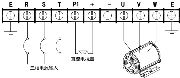
g) 132KW-315KW 变频器主回路端子台配线图 (如图 3-3g)
