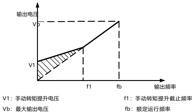
图 6-5 手动转矩提升示意图
