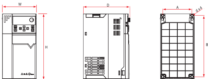
图8-3 ××××0.7GB~××××T185G外型尺寸及安装尺寸示意图
