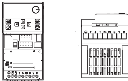
图3-3 ××××T0.7G(B)~××××T55G(B)主回路端子分布图
