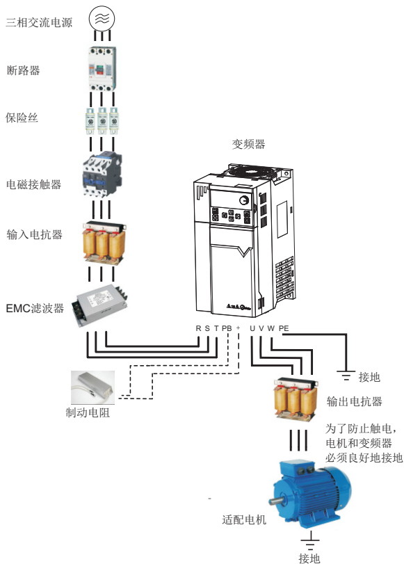
图2-1 系统构成
