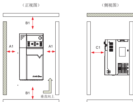
图3-1 单台机器 安装空间
