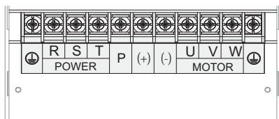
图3-4 ××××T75G~××××T185G主回路端子分布图
